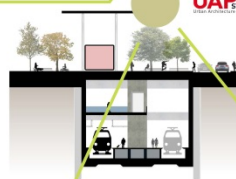
.sezione trasversale E_1:100
